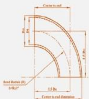
b. Long Radius Elbow
